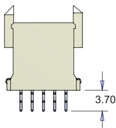
NO SHIELD 71-AB25V-000-11XX
