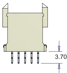
NO SHIELD 71-AB19V-000-11XX
