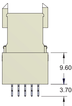
STAND-OFF, NO SHIELD 71-AB19V-020-11-XX
