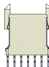
SHIELD BOTH SIDE 71-AB19V-300-11XX
