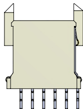
SHIELD F PIN SIDE 71-AB19V-100-11XX
