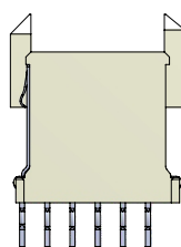
SHIELD Z PIN SIDE 71-AB19V-200-11XX
