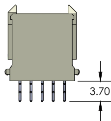
NO SHIELD 71-A25V-000-11XX
