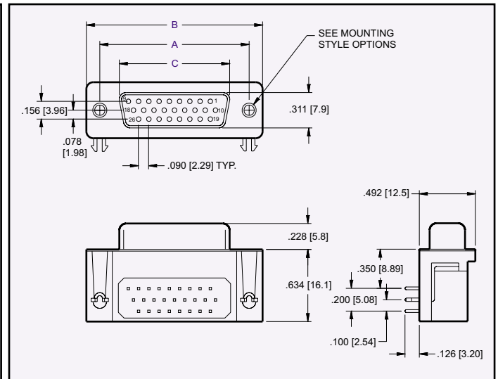
RECEPTACLE
